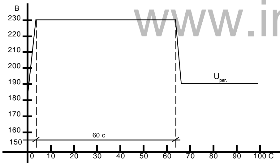
Рисунок 13 - График изменения выходного напряжения стабилизатора в режиме регулятора светового потока
