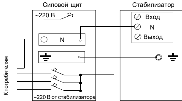
Рисунок 2. Схема электрических соединений
