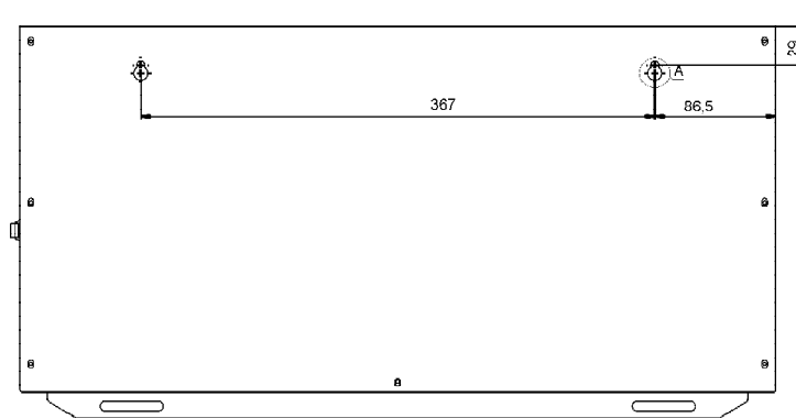
Габаритные и установочные размеры стабилизатора напряжения переменного тока LIDER PS3000W-50
