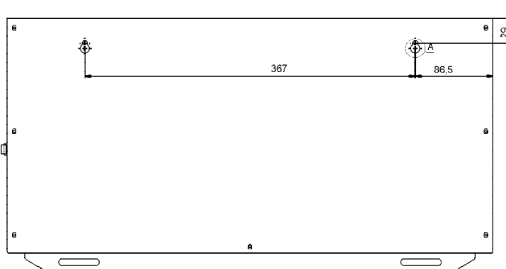
Габаритные и установочные размеры стабилизатора напряжения переменного тока LIDER PS3000W-30
