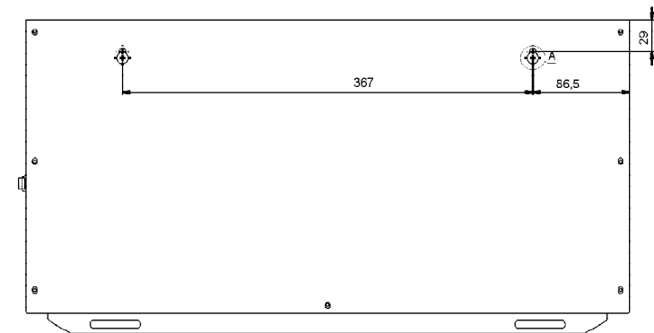
Габаритные и установочные размеры стабилизатора напряжения переменного тока LIDER PS3000SQ-25
